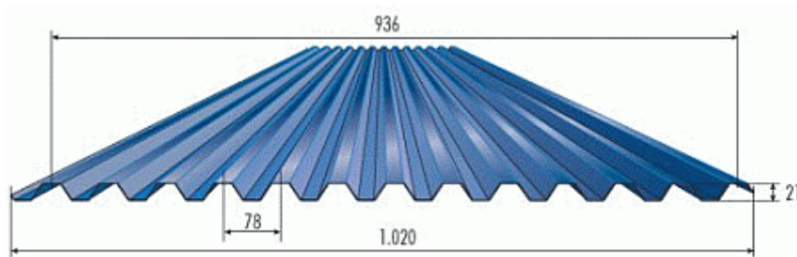
Profilo grecato Alubel 21 - sezione trasversale
